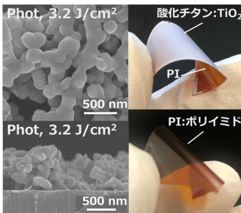
ポリイミドへの酸化チタン膜の形成 T. Sugahara et al., ACS. Appl. Ele. Mater., 2, 6, 1670 (2020).
